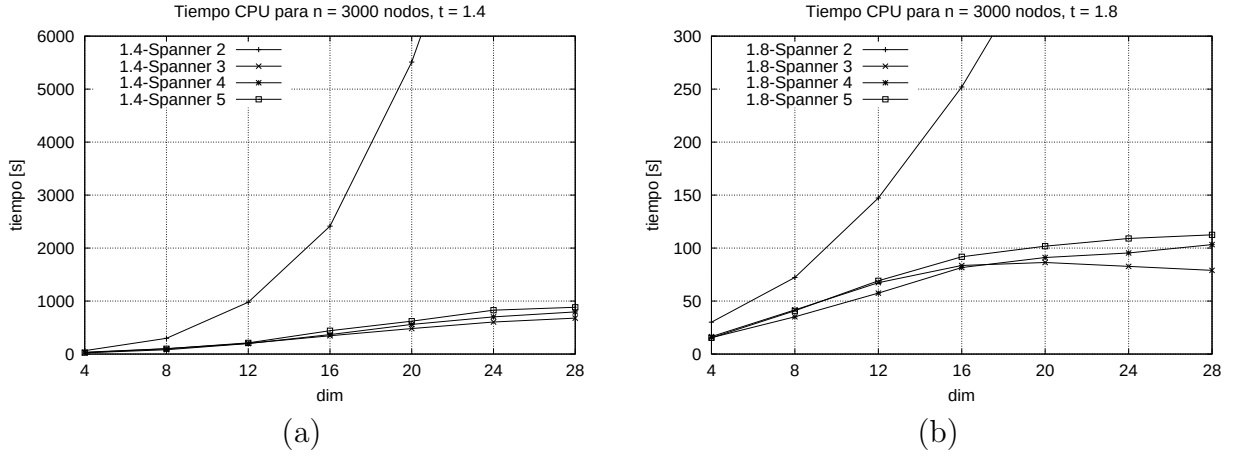
Figura 6.3: Tiempo de CPU para n = 3000 variando la dimensión. En (a) t -Spanner2 alcanza 14000 segundos en dim = 28 . En (b) t -Spanner2 alcanza 600 segundos en dim = 28 .
