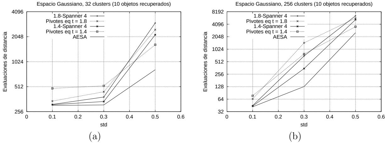
Figura 6.21: Consultas por rango en espacios vectoriales gaussianos, en promedio se recuperan 10 objetos por consulta.
