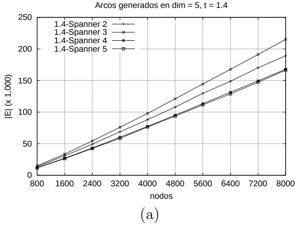
Figura 6.6: Arcos generados para dim = 5 variando la cantidad de nodos.
