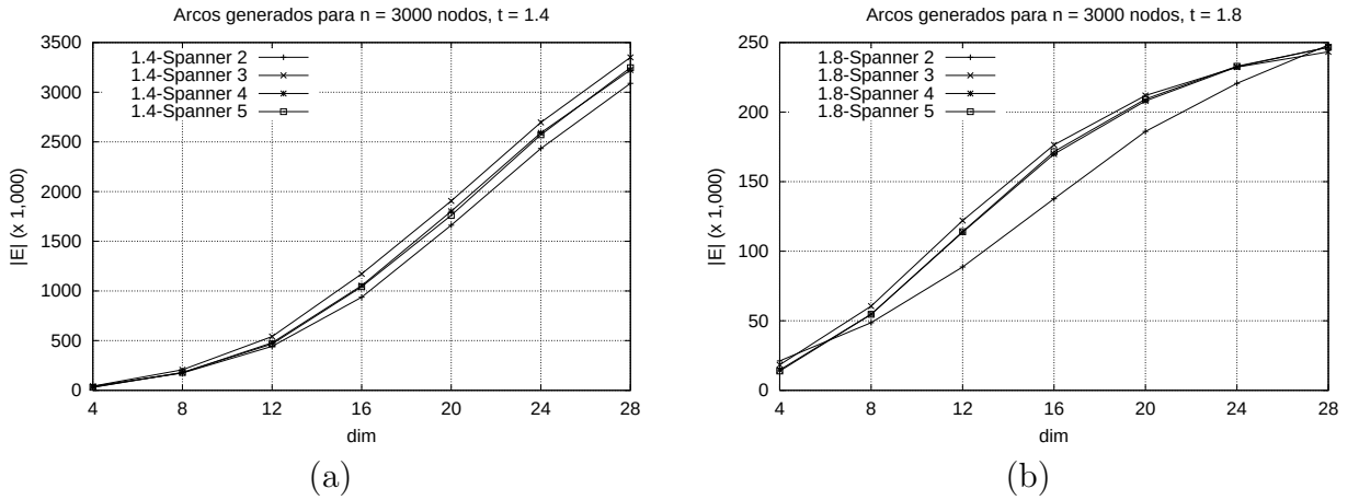
Figura 6.4: Arcos generados para n = 3000 variando la dimensión.
