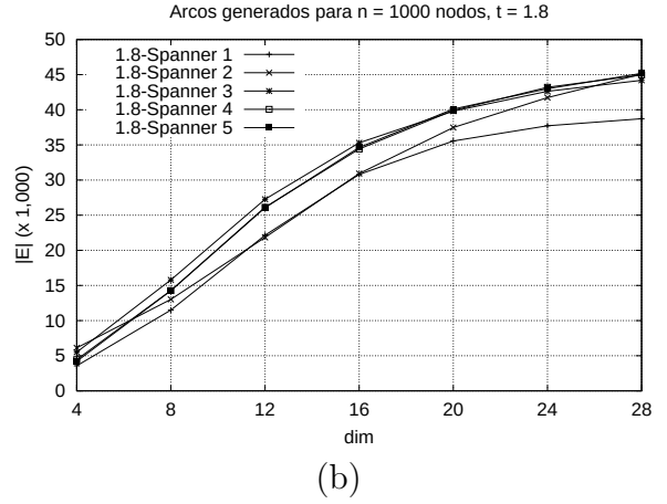
Figura 6.2: Comparación inicial de arcos generados para los cinco algoritmos. La cantidad de elementos es n = 1000 .
