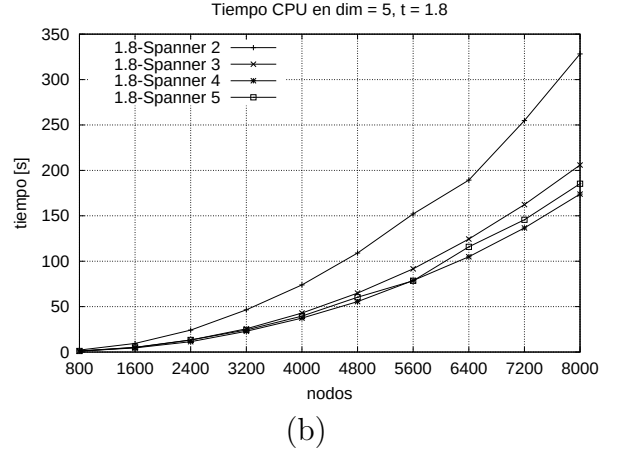
Figura 6.5: Tiempo de CPU para dim = 5 variando la cantidad de nodos.
