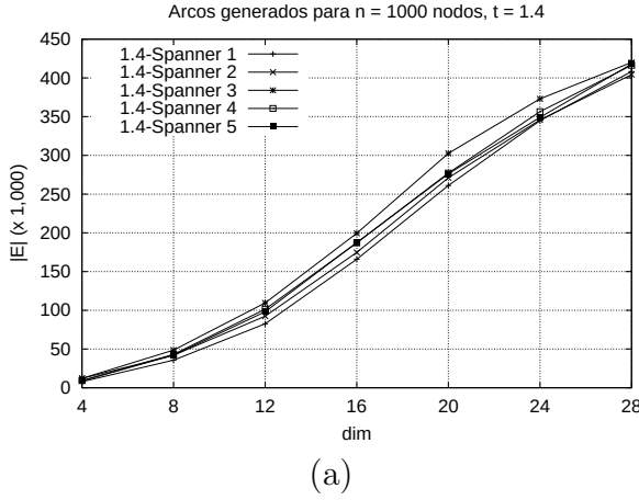
Figura 6.2: Comparación inicial de arcos generados para los cinco algoritmos. La cantidad de elementos es n = 1000 .
