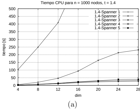
Figura 6.1: Comparación inicial de tiempos para los cinco algoritmos. La cantidad de elementos es n = 1000 . En (a) t -Spanner1 alcanza 2500 segundos en dim = 28 . En (b) t -Spanner1 alcanza 250 segundos en dim = 28 .
