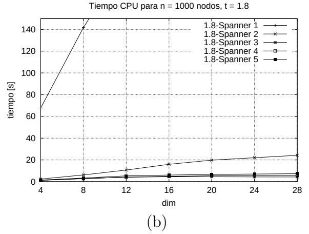
Figura 6.1: Comparación inicial de tiempos para los cinco algoritmos. La cantidad de elementos es n = 1000 . En (a) t -Spanner1 alcanza 2500 segundos en dim = 28 . En (b) t -Spanner1 alcanza 250 segundos en dim = 28 .
