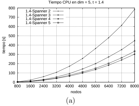
Figura 6.5: Tiempo de CPU para dim = 5 variando la cantidad de nodos.
