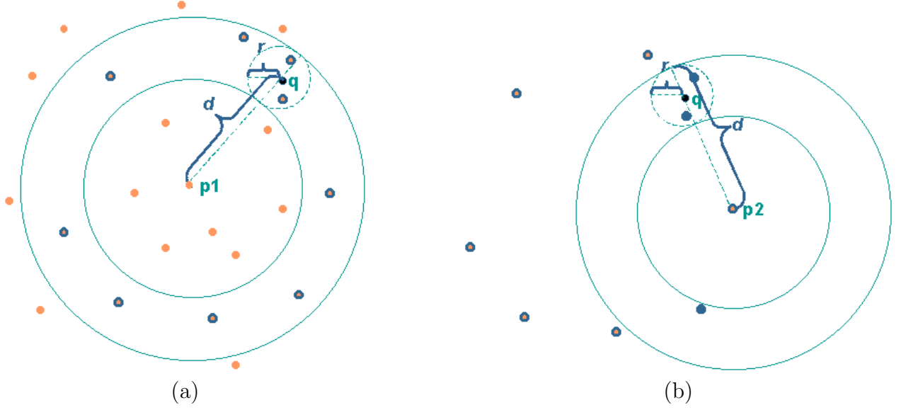
Figura 2.2: Ejemplo de AESA.
