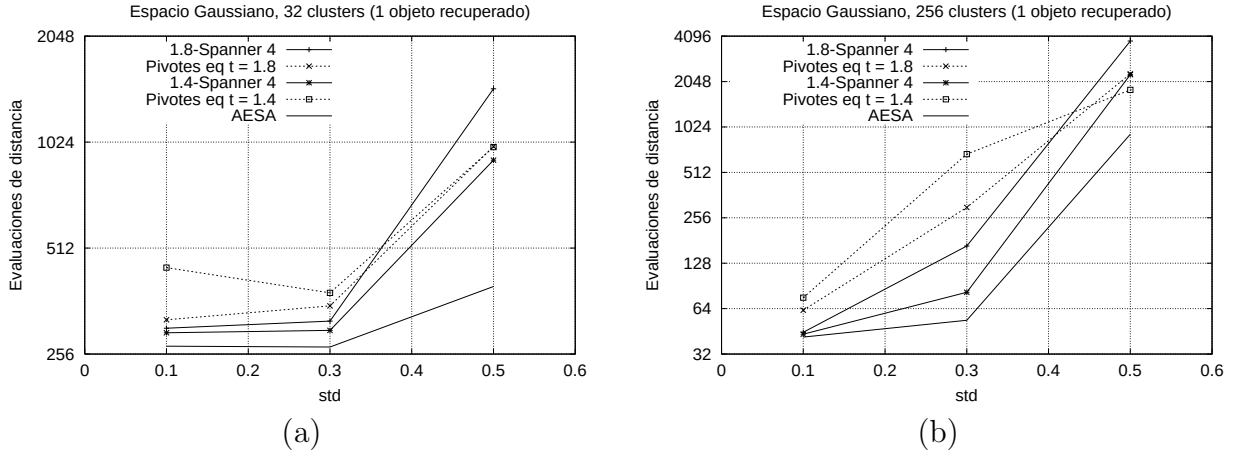
Figura 6.20: Consultas por rango en espacios vectoriales gaussianos, en promedio se recupera 1 objeto por consulta.
