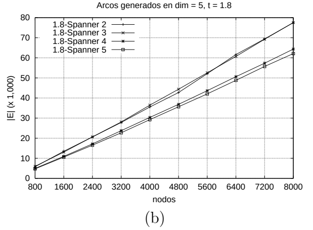
Figura 6.6: Arcos generados para dim = 5 variando la cantidad de nodos.
