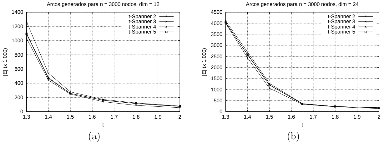
Figura 6.8: Arcos generados para n = 3000 variando t .
