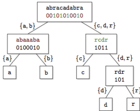
Figura 2.1: Ejemplo de un wavelet tree de la palabra abracadabra . Figura sacada de https://en.wikipedia.org/wiki/File:Wavelet_tree.png
